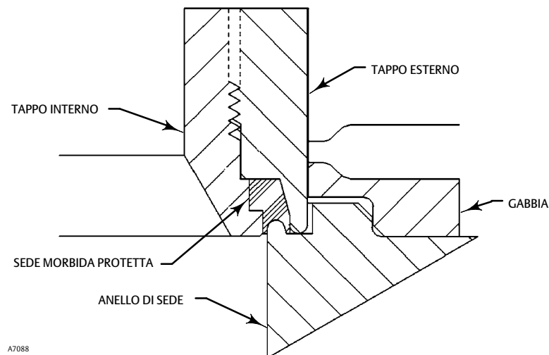
Figura 6. TSO (chiusura a tenuta stagna), dettaglio della sede morbida protetta
