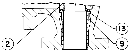
DETTAGLIO DI EAT CON RIVESTIMENTO (SOLO SEDE METALLICA)
