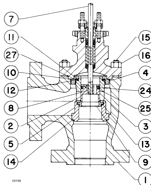
EAT CON ANELLO DI SEDE METALLICO
