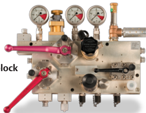
Umschaltpanel
