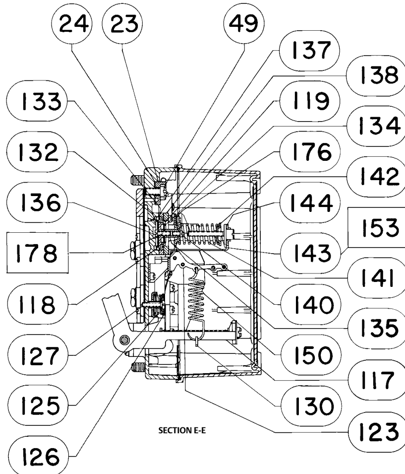
Figure 26. Ensemble positionneurs (suite)
