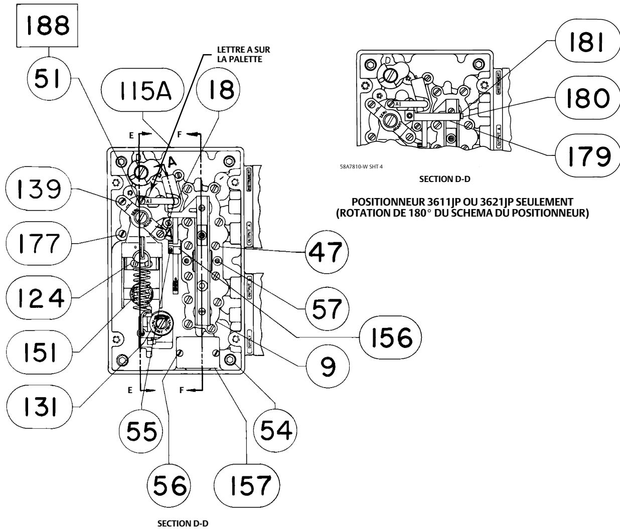
Figure 26. Ensemble positionneurs
