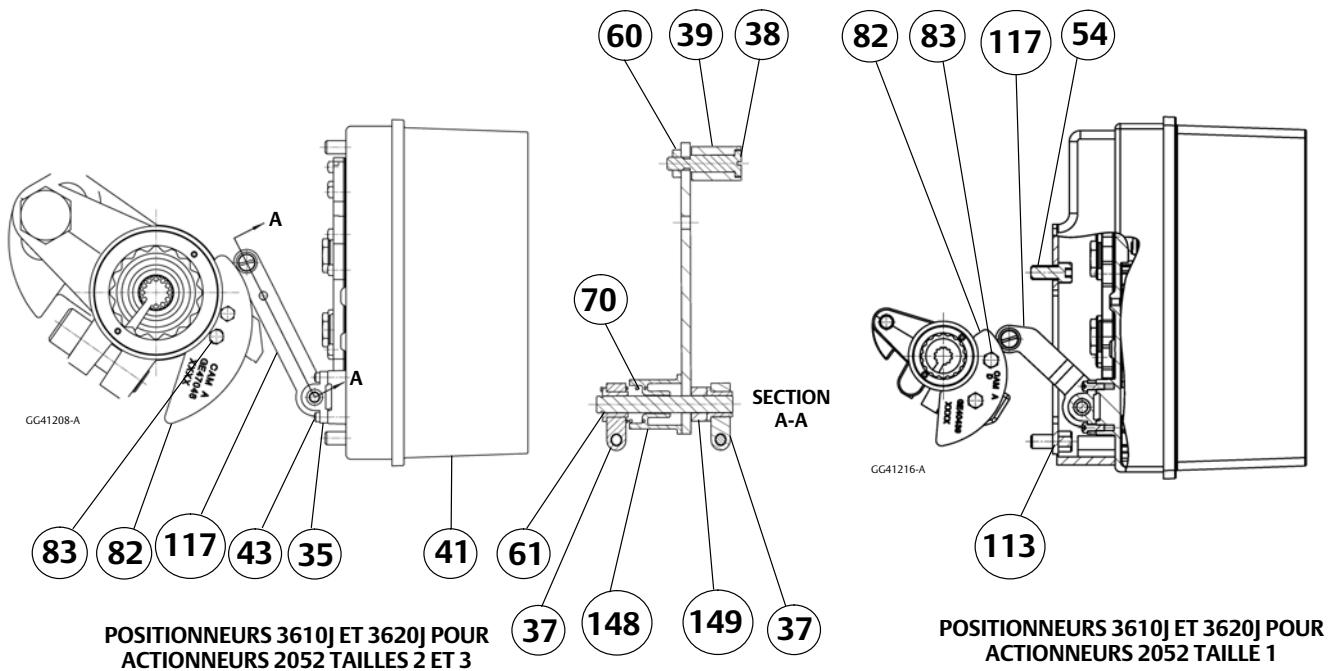
Figure 29. Dispositifs de contre-réaction pour positionneurs 3610J, 3610JP, 3620J et 3620JP de Fisher (suite)
