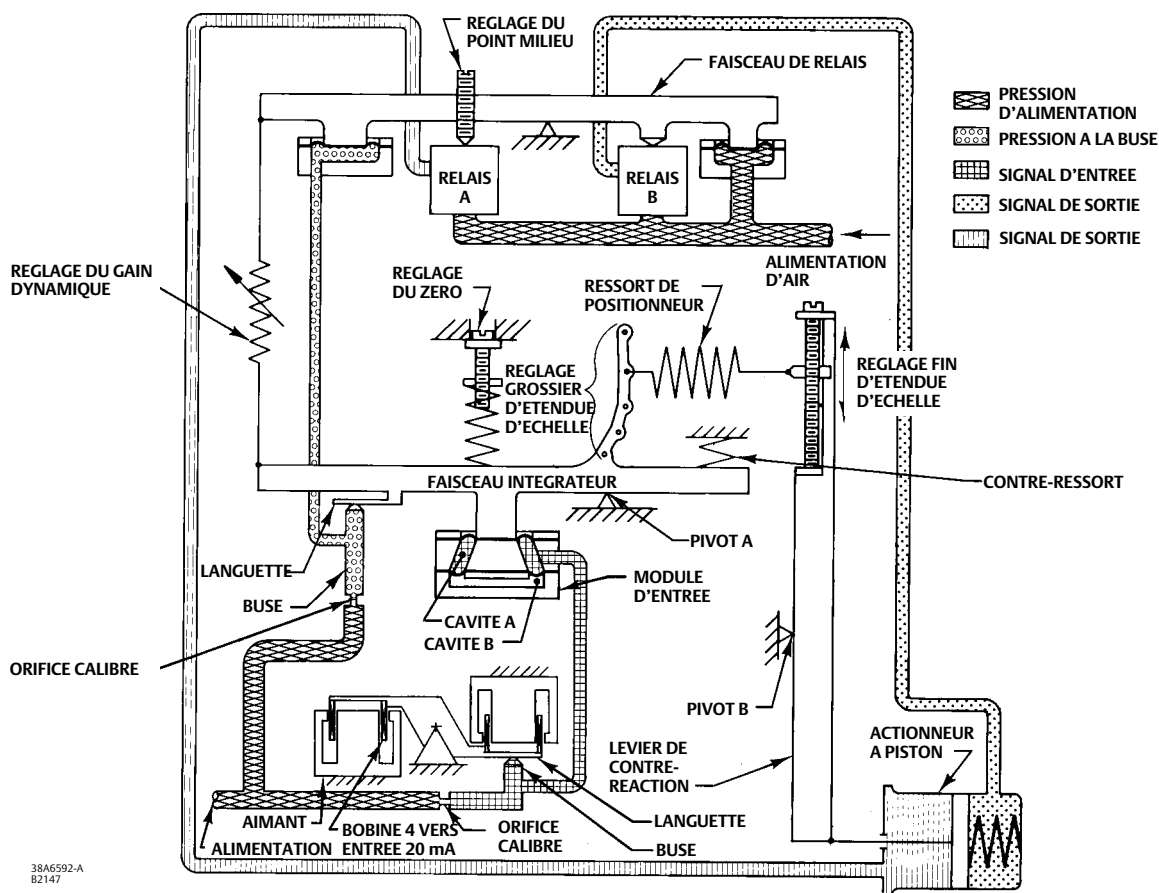
Figure 25. Schéma d'un positionneur 3621JP de Fisher
