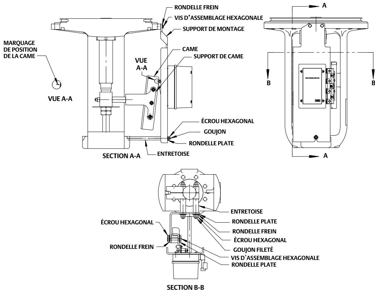
Figure 7. Montage typique des positionneurs 3610JP et 3620JP de Fisher sur des actionneurs à tige coulissante à longue course
