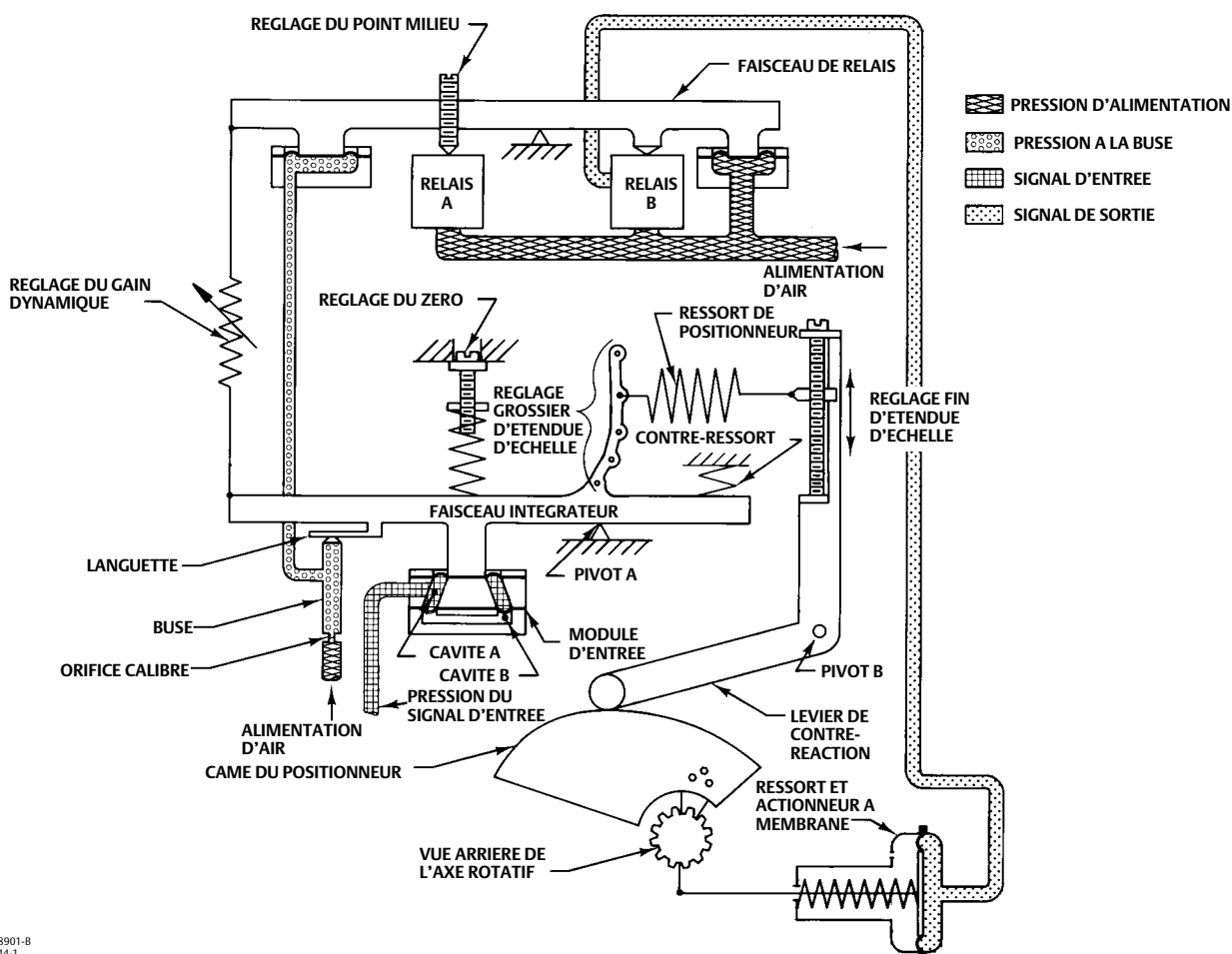
Figure 20. Schéma d'un positionneur 3610J de Fisher
