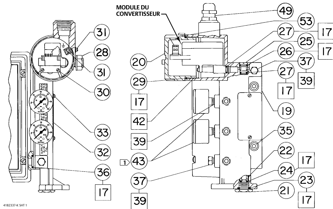
Figure 31. Ensemble convertisseur électropneumatique Type 3622
