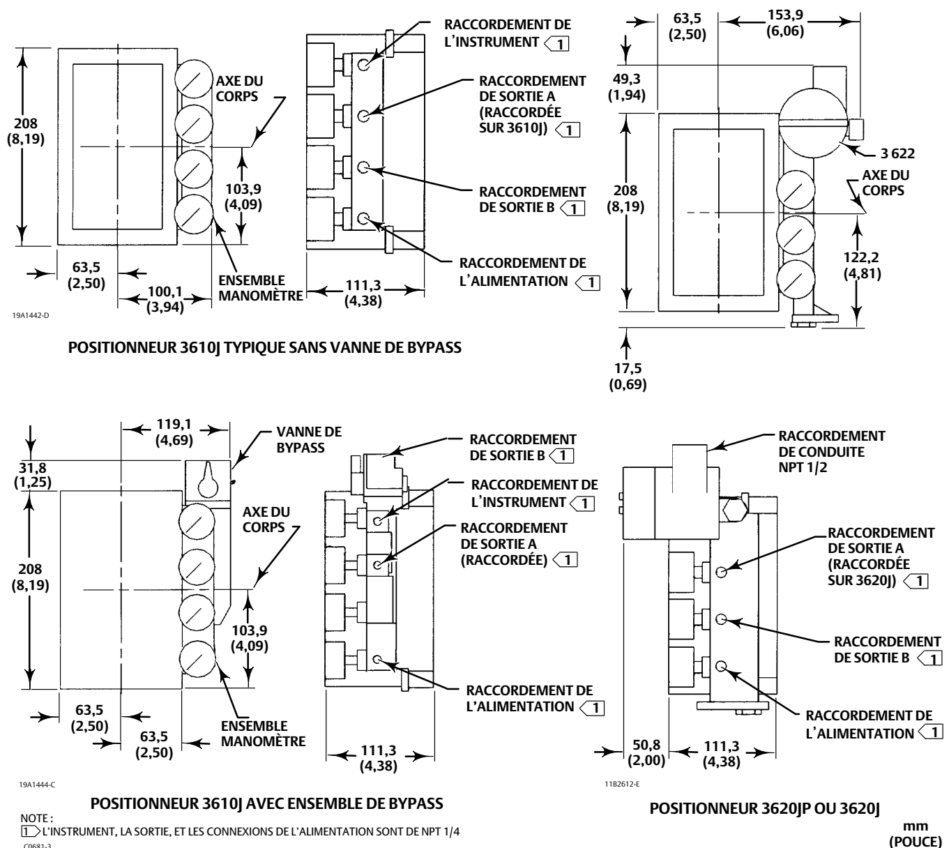
Figure 9. Raccordements et dimensions de montage typiques
