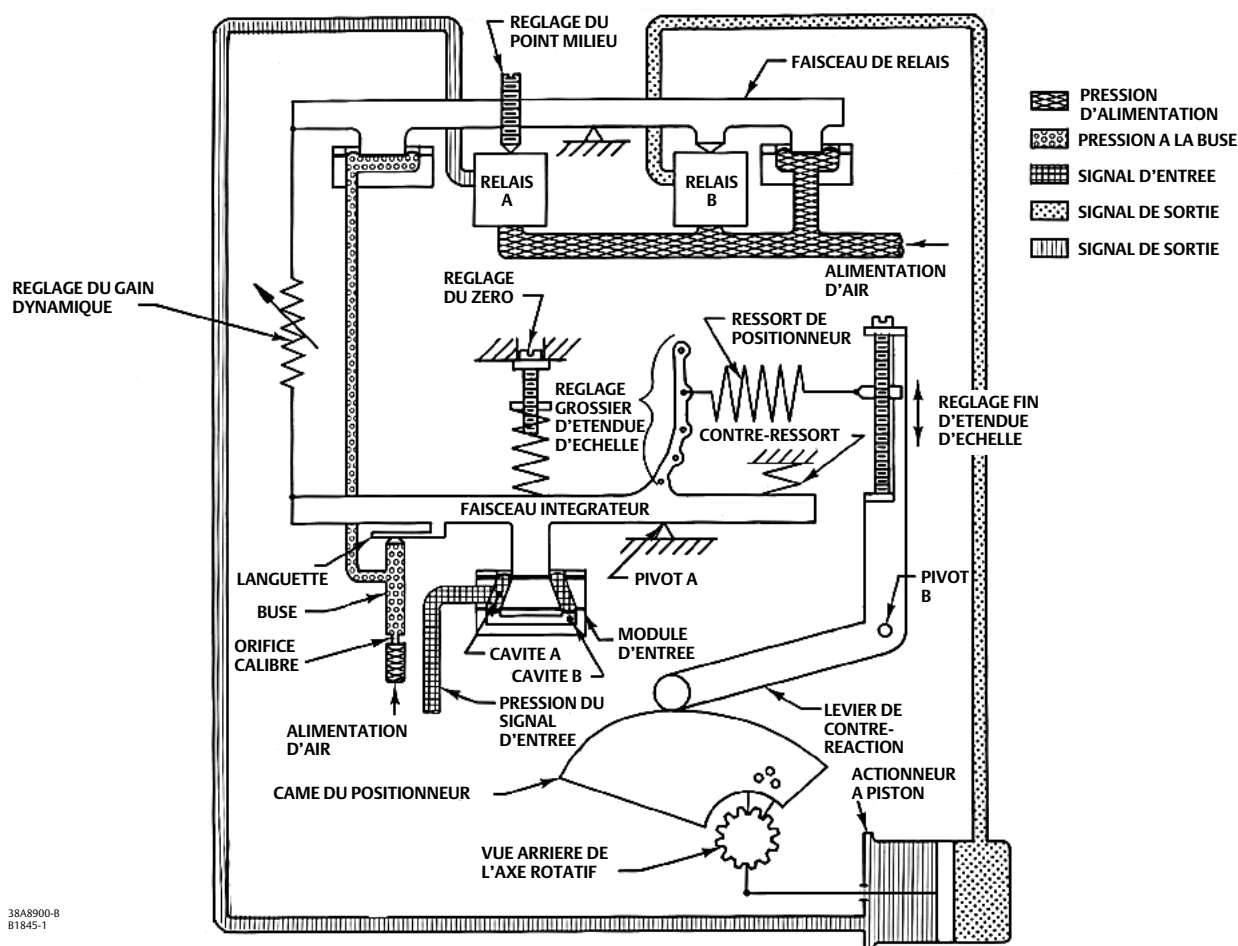
Figure 21. Schéma d'un positionneur 3610JP de Fisher
