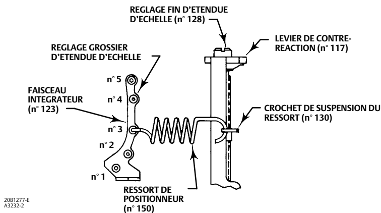
Figure 16. Etendue d'échelle
