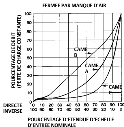
Figure 18. Caractéristiques de débit de cames diverses lorsqu'elles sont utilisées avec une vanne à clapet à pourcentage égal, vanne fermée par manque d'air
