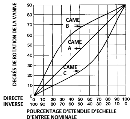
Figure 19. Caractéristiques de débit de cames diverses lorsqu'elles sont utilisées avec une vanne à clapet à pourcentage égal, vanne ouverte par manque d'air
