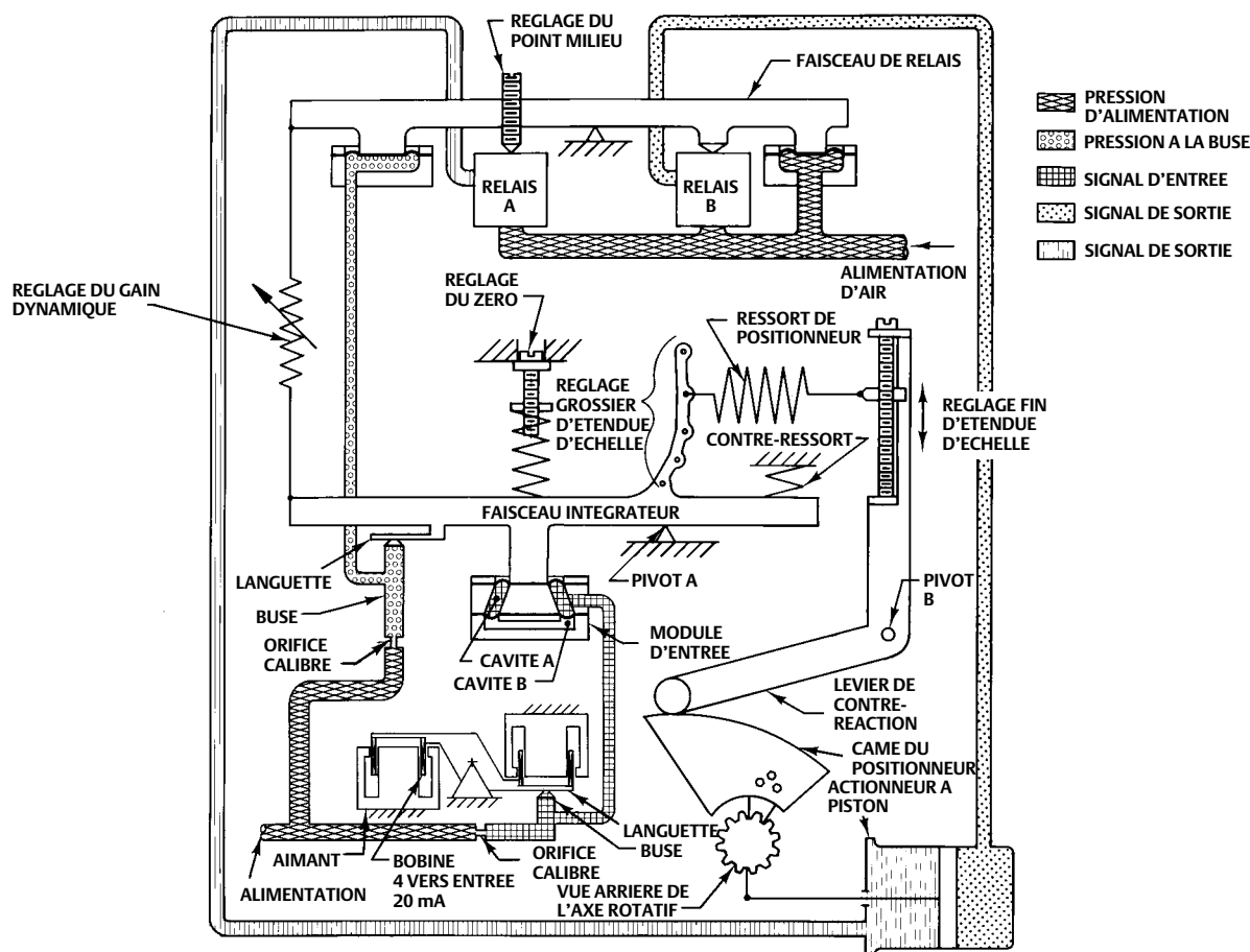
Figure 24. Schéma d'un positionneur 3620JP de Fisher
