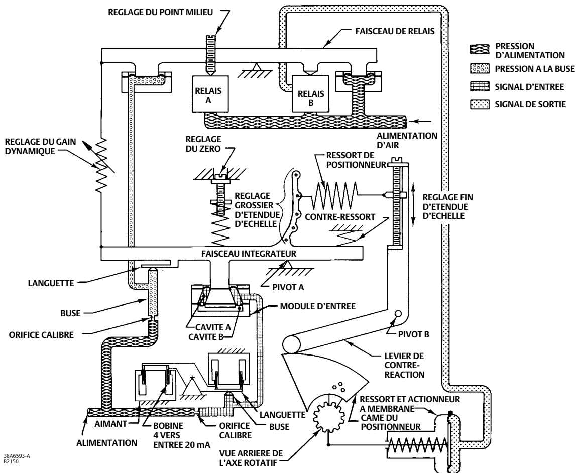
Figure 23. Schéma d'un positionneur 3620J de Fisher
