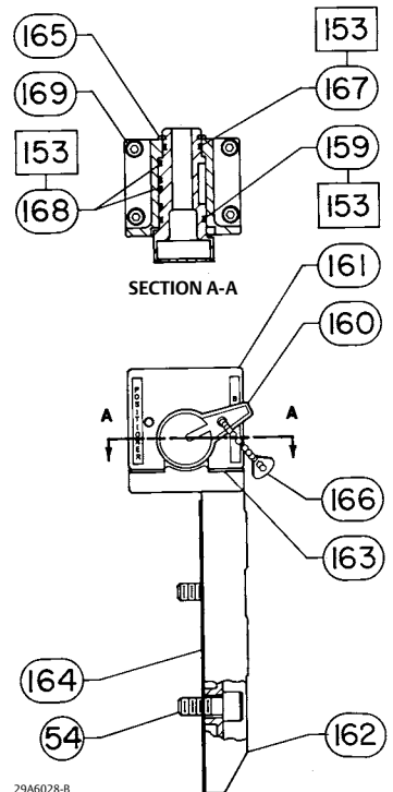
ENSEMBLE VANNE DE DERIVATION POUR POSITIONNEURS 3610J
