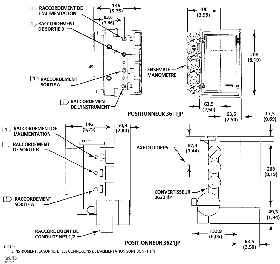
Figure 9. Raccordements et dimensions de montage typiques (suite)
