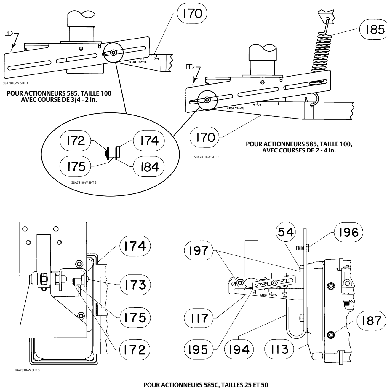
Figure 30. Dispositifs de contre-réaction pour positionneurs 3611JP et 3621JP de Fisher
