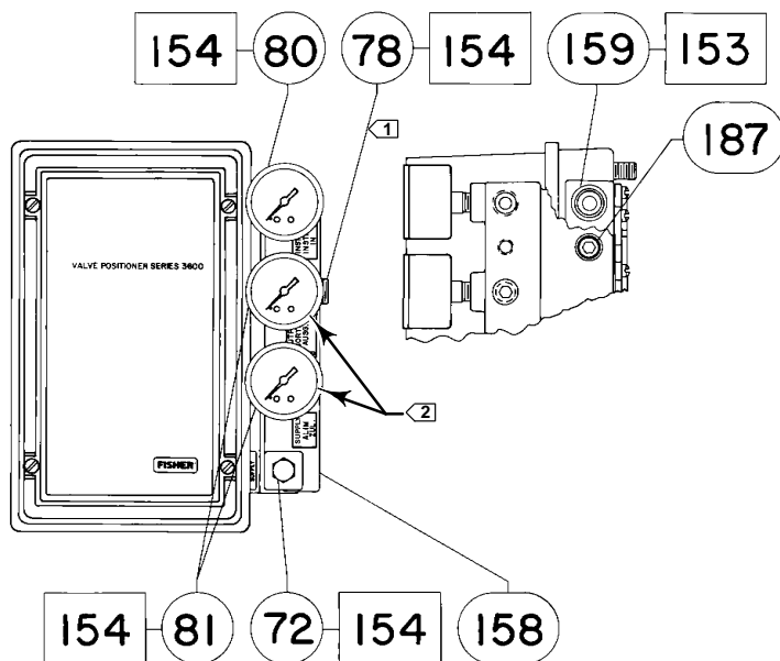
Figure 27. Ensembles manomètre et vanne de dérivation
