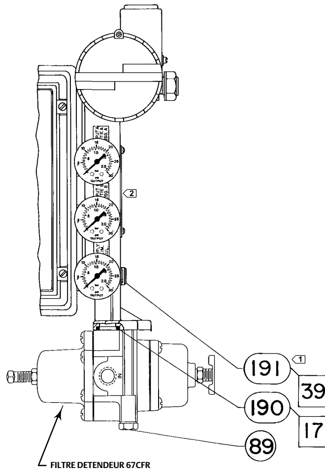
Figure 28. Positionneur 3620J à filtre détenteur intégré de Fisher
