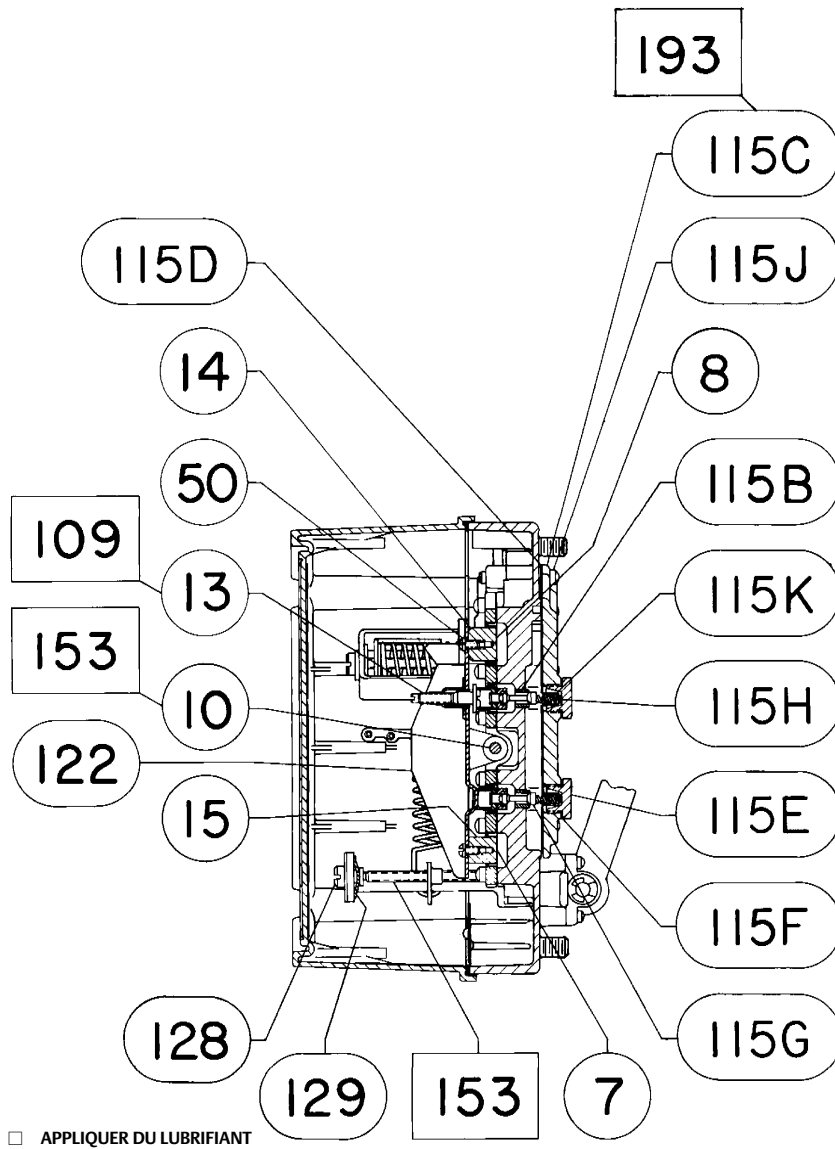
Figure 26. Ensemble positionneurs (suite)
