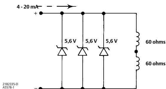
Figure 12. Circuit équivalent du convertisseur 3622 de Fisher
