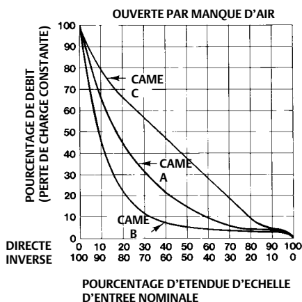
Figure 19. Caractéristiques de débit de cames diverses lorsqu'elles sont utilisées avec une vanne à clapet à pourcentage égal, vanne ouverte par manque d'air
