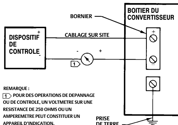
Figure 13. Schéma de câblage sur site typique
