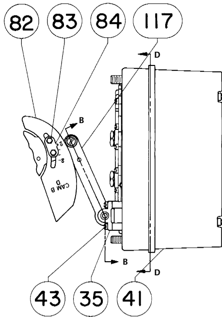
Figure 29. Dispositifs de contre-réaction pour positionneurs 3610J, 3610JP, 3620J et 3620JP de Fisher
