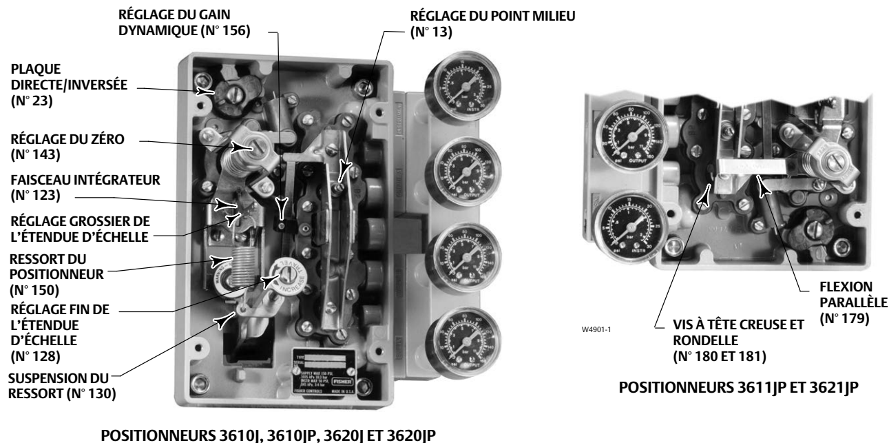
Figure 14. Réglages de l'étalonnage
