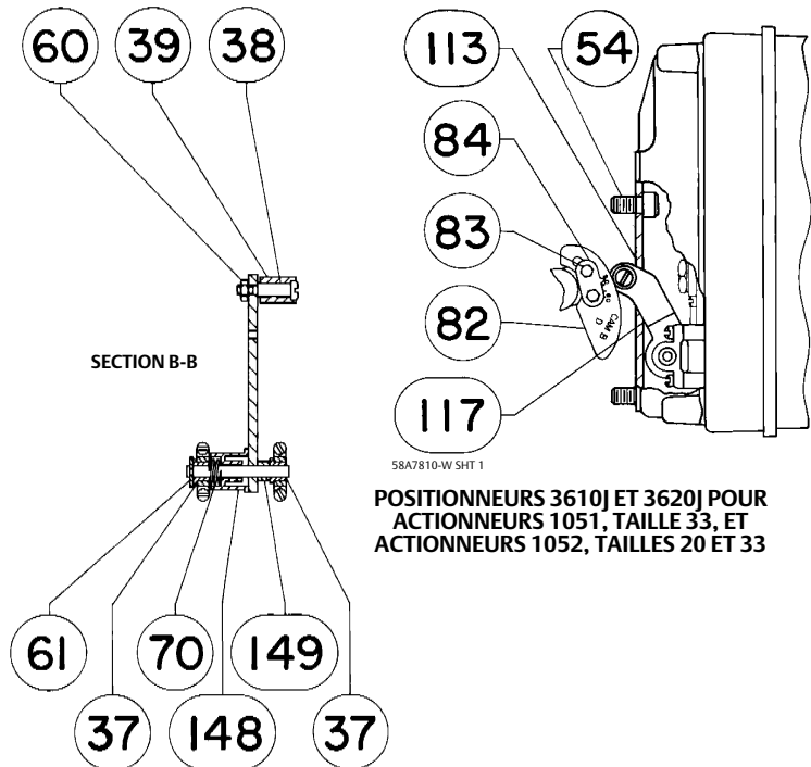
Figure 29. Dispositifs de contre-réaction pour positionneurs 3610J, 3610JP, 3620J et 3620JP de Fisher
