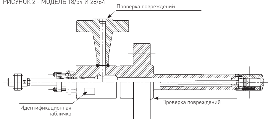
РИСУНОК 2 - МОДЕЛЬ 18/54 И 28/64
