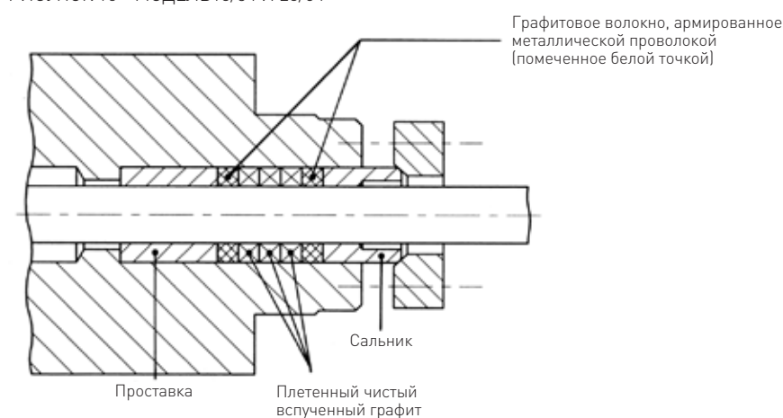
РИСУНОК 10 - МОДЕЛЬ 18/54 И 28/64
