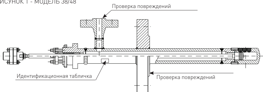
РИСУНОК 1 - МОДЕЛЬ 38/48
