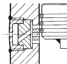
ДЕТАЛЬ 'А'
