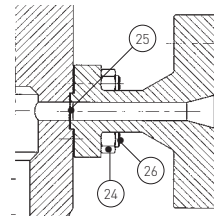
** ДЕТАЛЬ 'В'
