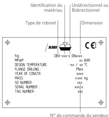
PLAQUE D'IDENTIFICATION
