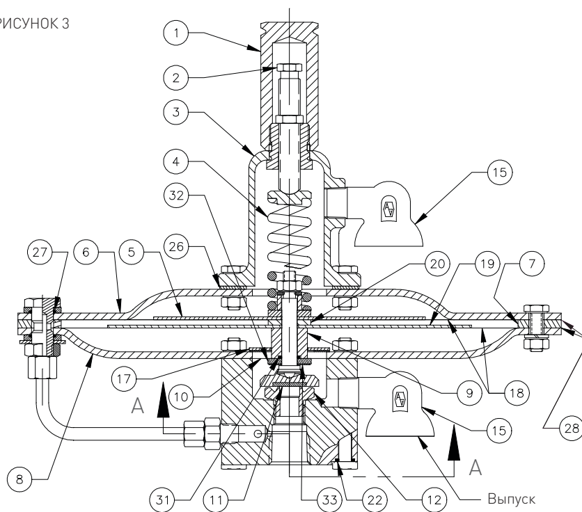
Серия 93 (Резиновое седло)
