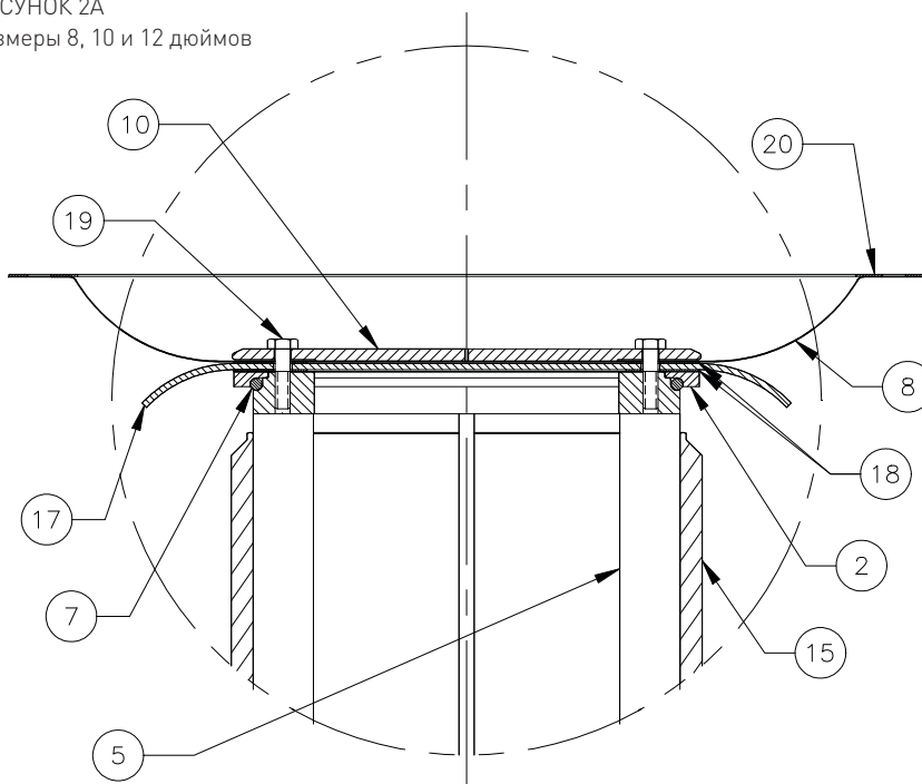
Мембрана из ПТФЭ с отражателем
