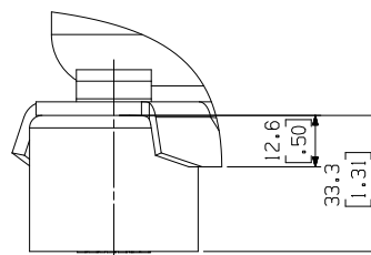
DETAIL Y SCALE 3:2
