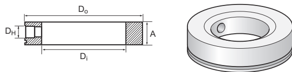
Abbildung 54: Spülringe
