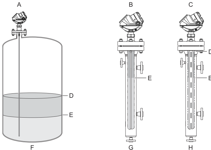
Abbildung 21: Messung der Trennschichthöhe
