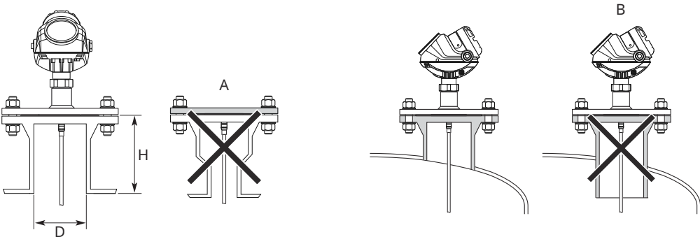
Abbildung 27: Montage in Stutzen
