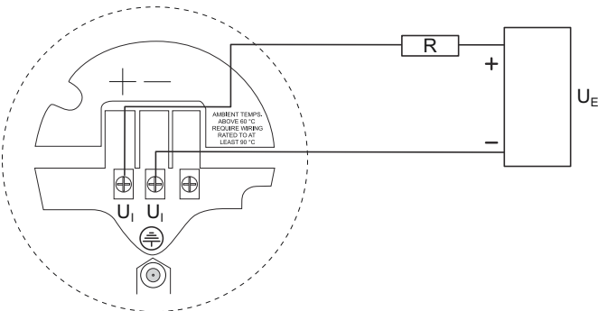
Abbildung 10: Externe Spannungsversorgung für HART
