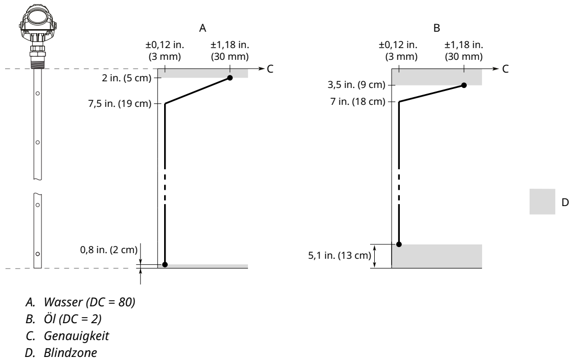
Abbildung 6: Genauigkeit über den Messbereich für Koaxialsonden
