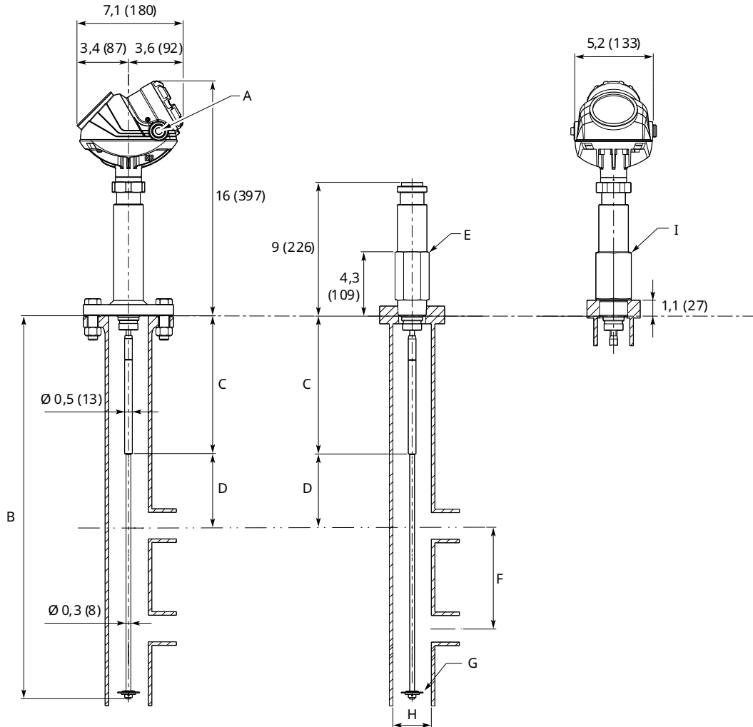
Abbildung 40: Starre Dampf-Einzelsonde für 2 in.-Bypass-Bezugsgefäß
