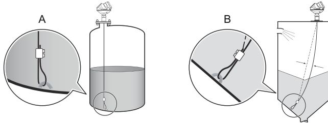
Abbildung 34: Stabilisieren der Sonde gegen Einwirkung seitlicher Kräfte
