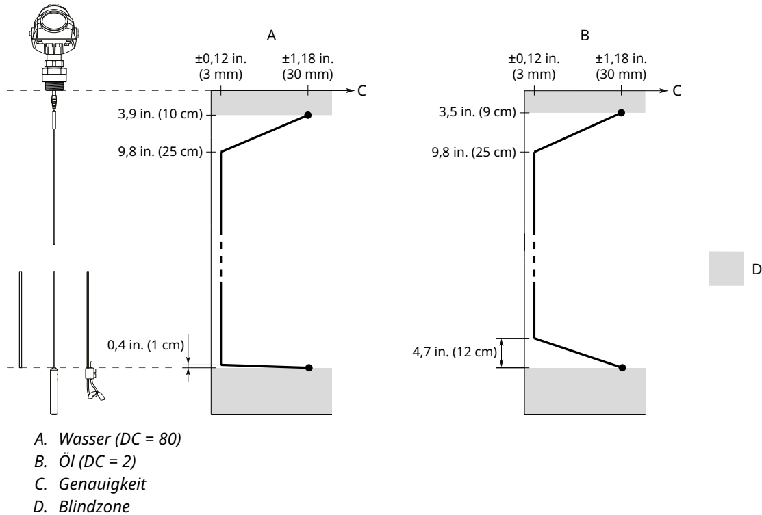
Abbildung 6: Genauigkeit über den Messbereich für Koaxialsonden
