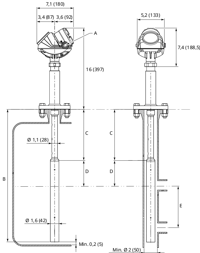
Abbildung 48: Integrierte Beruhigungsrohr-Dampfsonde für Bypass-Bezugsgefäß ab 3 in.
