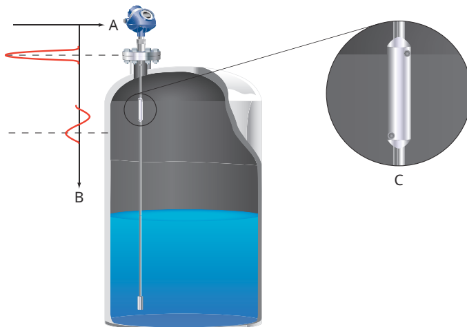
Abbildung 12: Verification Reflector
