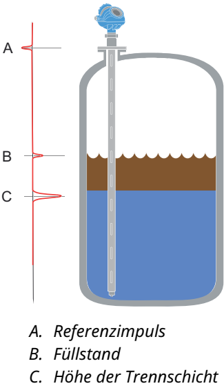
Abbildung 1: Messprinzip
