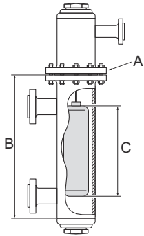
Abbildung 29: Vorhandenes Verdränger-Bezugsgefäß
