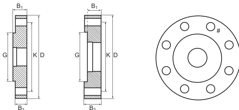
Abbildung 53: Herstellerspezifische Flansche
