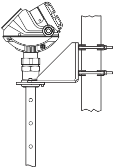
Abbildung 32: Koaxialsonde bei einer offenen Anwendung
