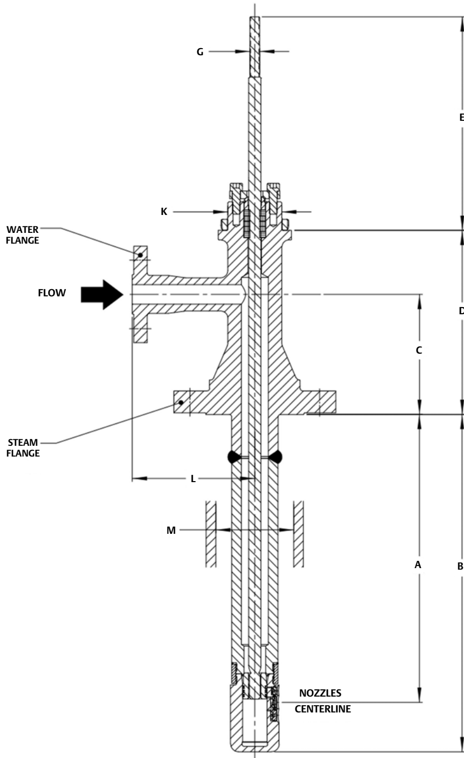
Figure 11. Yarway Templo 4300
