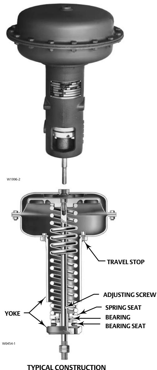
Fisher 656 Actuator
