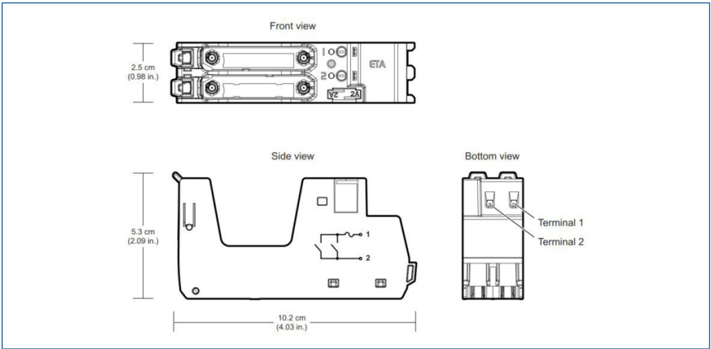
LS CHARM Redundant ETA Relay Terminal Block.
