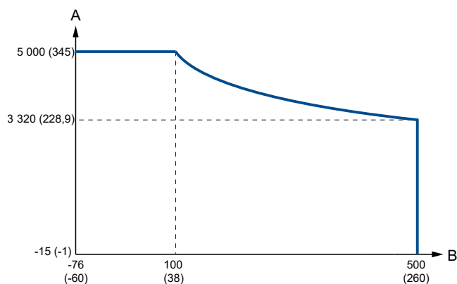
Illustration 16 : HP – Raccord de réservoir haute pression (Code P)
