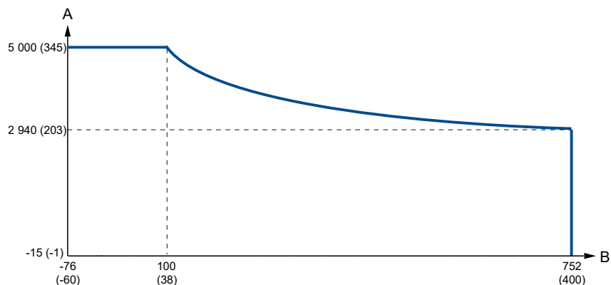
Illustration 15 : HTHP - Raccord de réservoir haute température et haute pression (code H)
