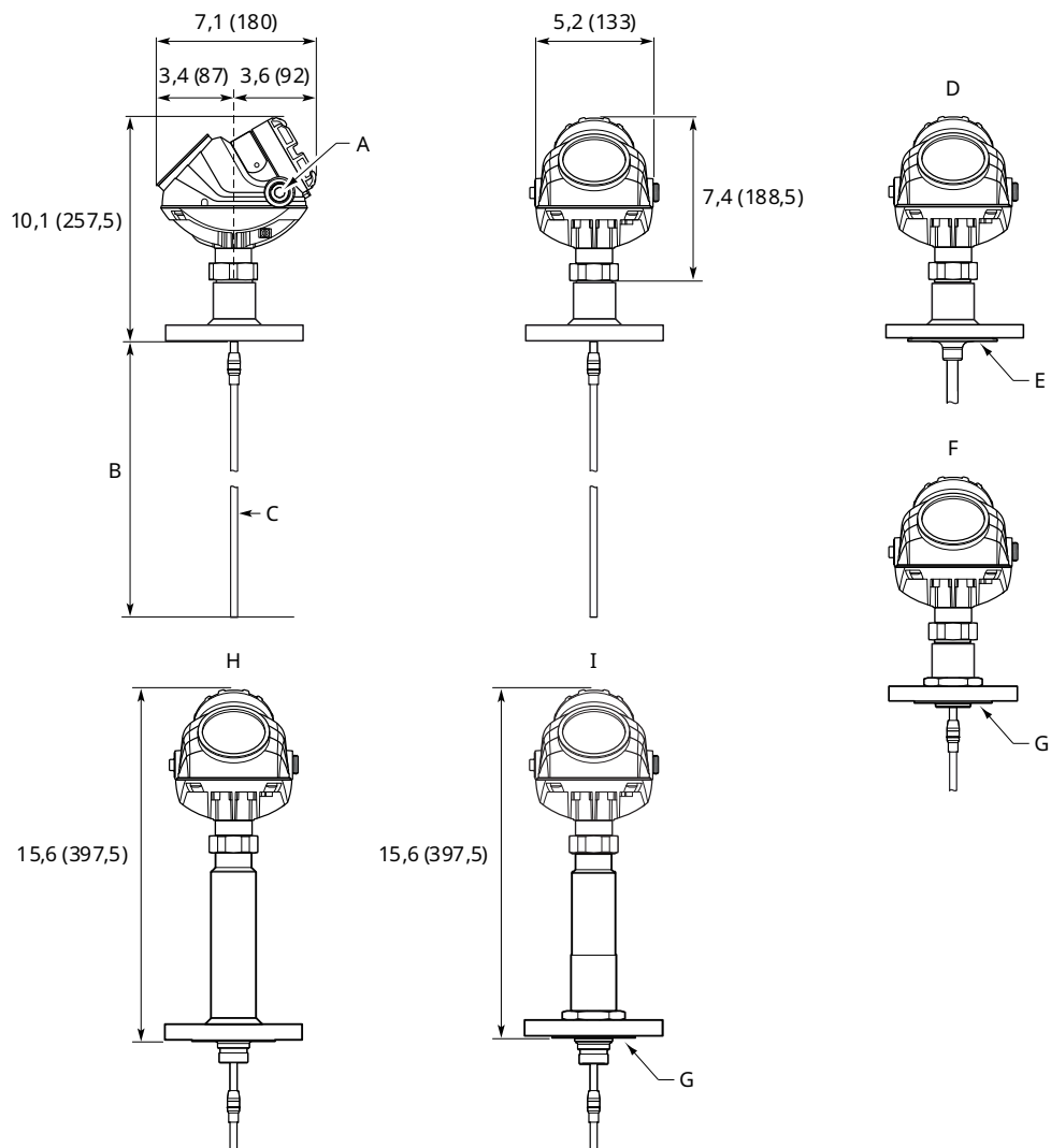
Illustration 35 : Sonde simple tige avec bride de raccordement
