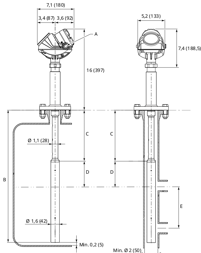
Illustration 48 : Sonde intégrée vapeur pour chambre de tranquillisation de 3 po et plus
