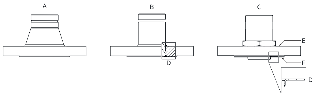
Illustration 52 : Raccordement à brides
