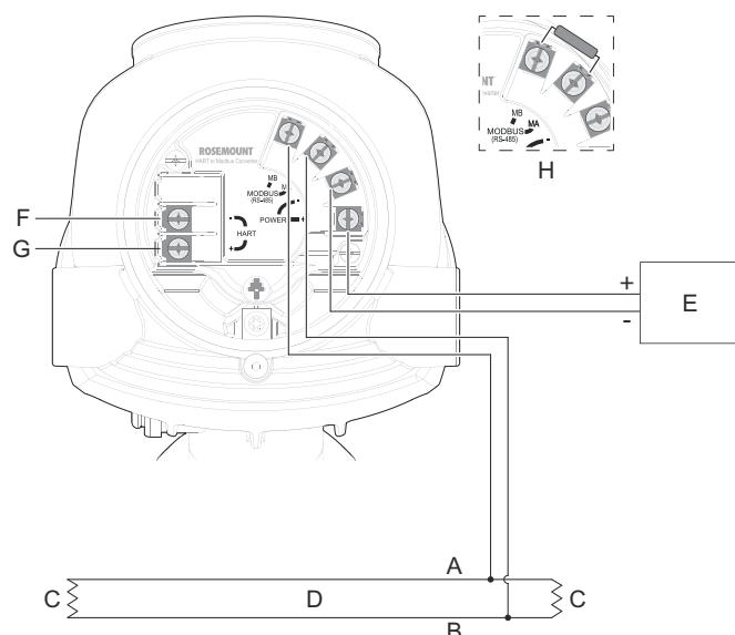
Illustration 11 : Schéma de câblage pour RS-485 avec Modbus®
