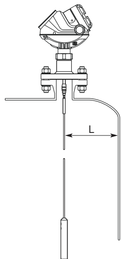
Illustration 26 : Exigence d'espace libre
