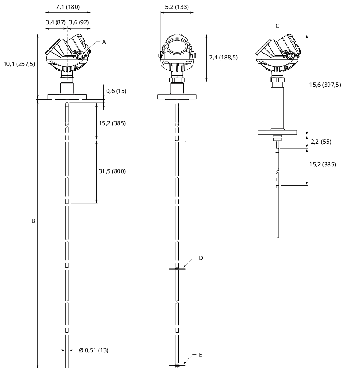
Illustration 38 : Sonde simple tige segmentée avec bride de raccordement
