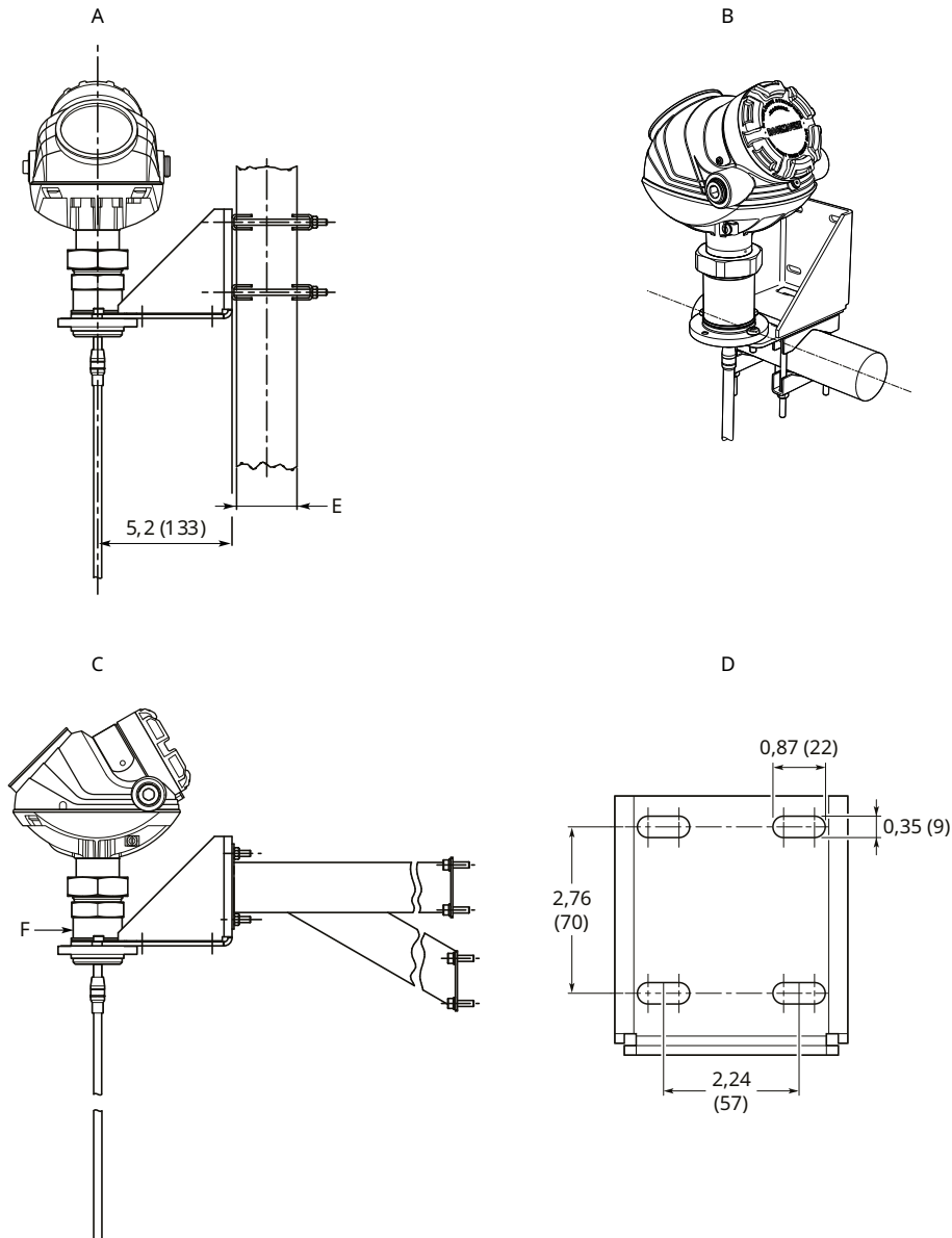
Illustration 49 : Support de montage (Code d'option BR)
