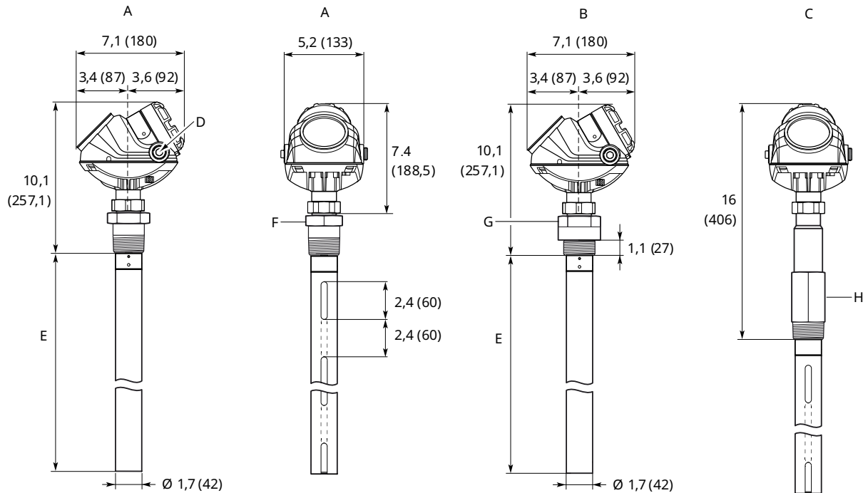
Illustration 47 : Grande sonde coaxiale avec raccordement fileté
