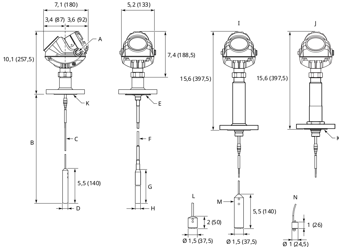
Illustration 41 : Sonde simple câble avec bride de raccordement
