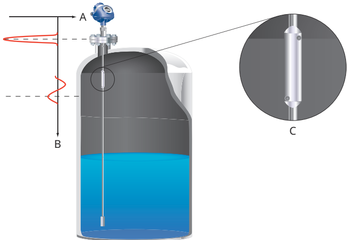
Illustration 12 : Réflecteur de vérification
