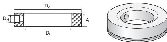
Illustration 54 : Bagues de raccord de rinçage
