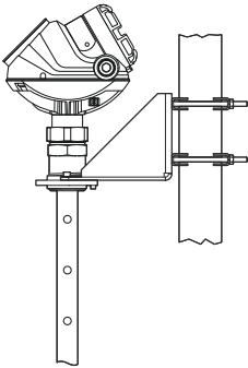
Illustration 32 : Sonde coaxiale dans une application en plein air
