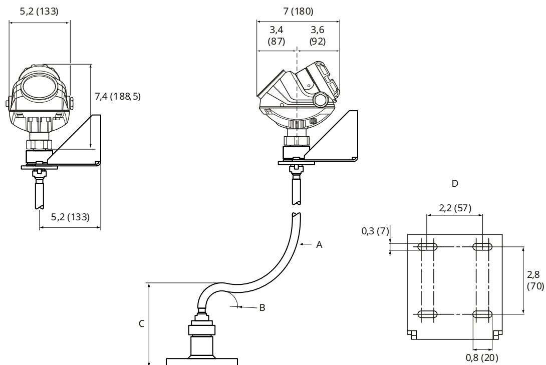
Illustration 50 : Boîtier déporté (code d'option B1, B2, B3)
