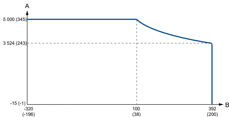
Illustration 17 : C - Raccord de réservoir à température cryogénique (code C)
