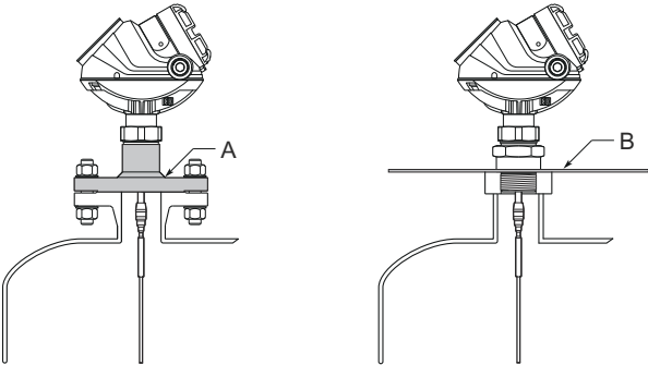
Illustration 33 : Montage dans des réservoirs non métalliques
