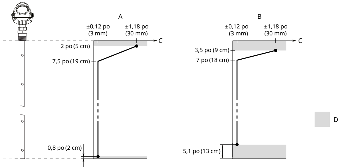
Illustration 6 : Précision sur la plage de mesure des sondes coaxiales
