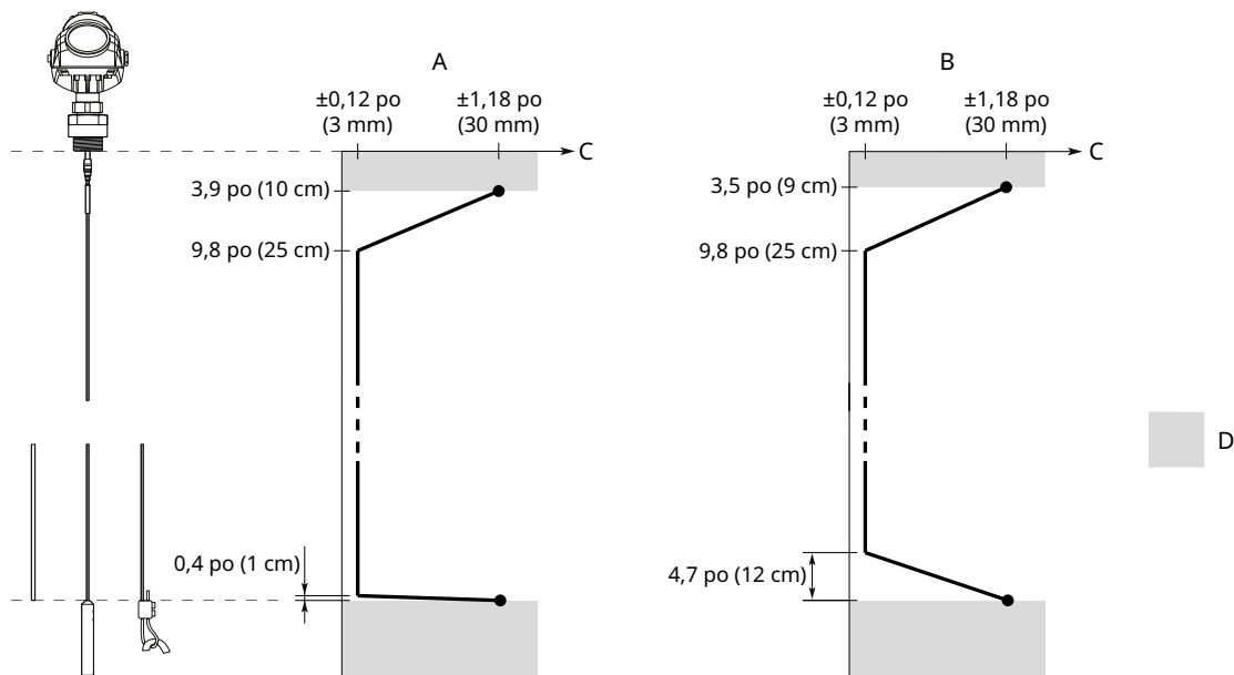
Illustration 5 : Précision sur la plage de mesure des sondes simple tige (tige/tige segmentée/câble)
