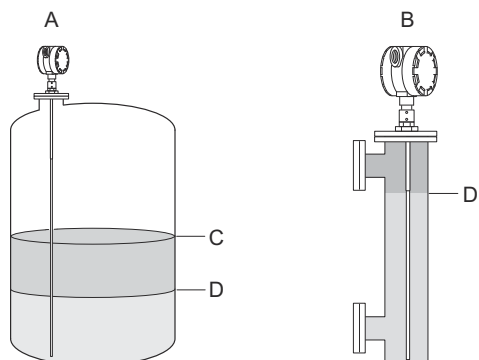
Illustration 11 : Mesure du niveau d'interface
