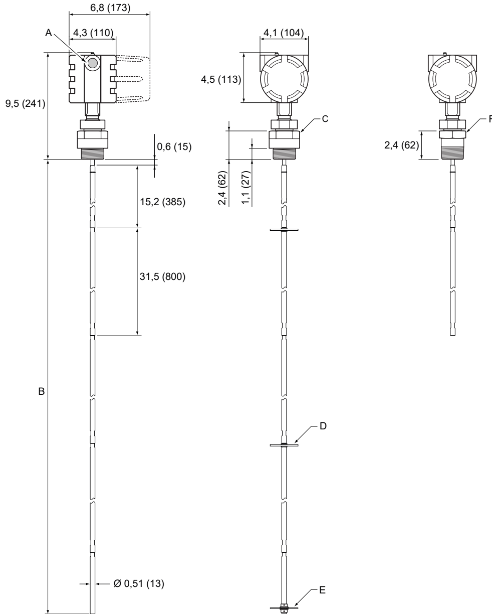
Illustration 25 : Sonde simple tige segmentée avec raccordement fileté
