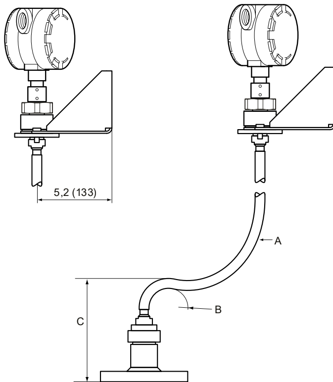
Illustration 31 : Boîtier déporté
