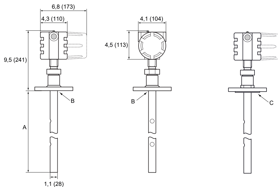
Illustration 28 : Sonde coaxiale avec bride de raccordement
