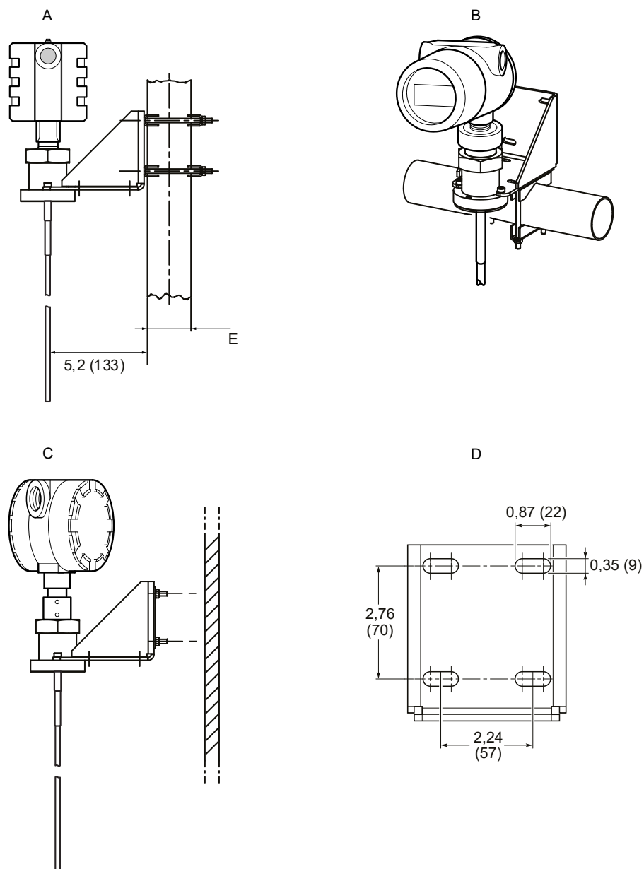
Illustration 30 : Montage sur support
