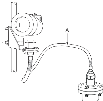
A. Câble de montage du boîtier déporté : 3, 6 ou 9 pi (1, 2 ou 3 m)
