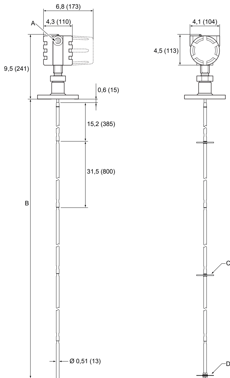
Illustration 24 : Sonde simple tige segmentée avec bride de raccordement
