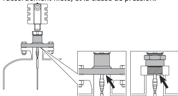
Illustration 9 : Valeur nominale maximale, raccords de réservoir standard
