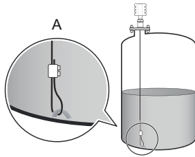
A. Sonde simple câble avec mandrin.
