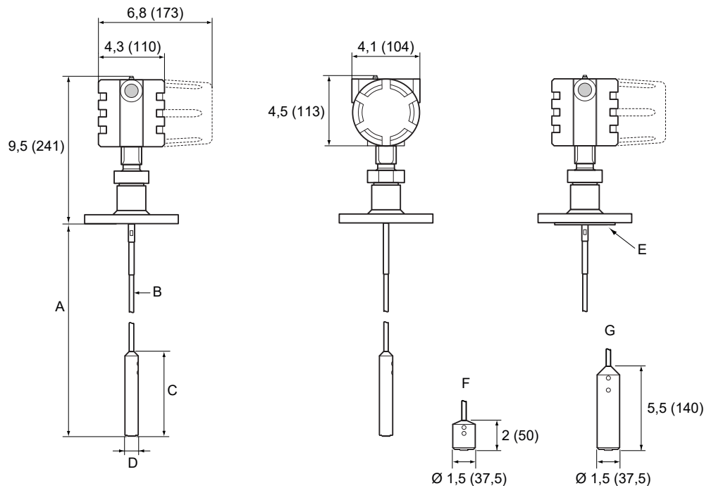
Illustration 26 : Sonde simple câble avec bride de raccordement
