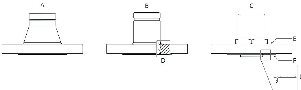
Illustration 32 : Raccordement à brides
