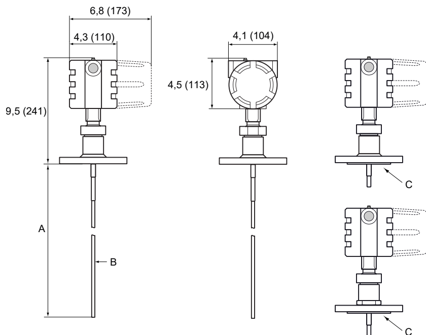
Illustration 22 : Sonde simple tige avec bride de raccordement
