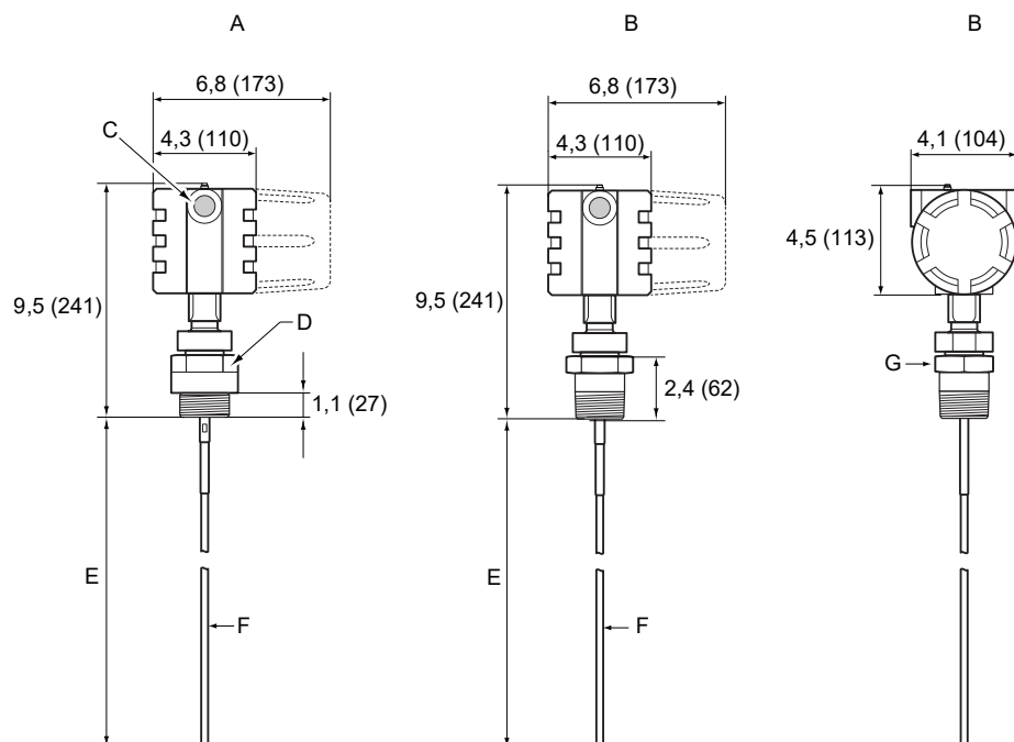
Illustration 23 : Sonde simple tige avec raccord fileté
