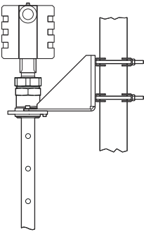
Illustration 19 : Sonde coaxiale dans une application en plein air
