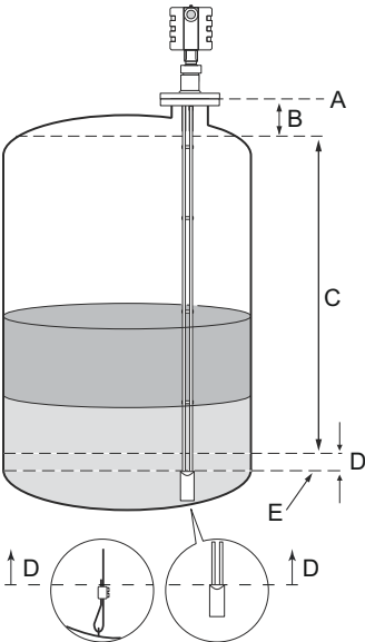
Illustration 3 : Zones de transition
