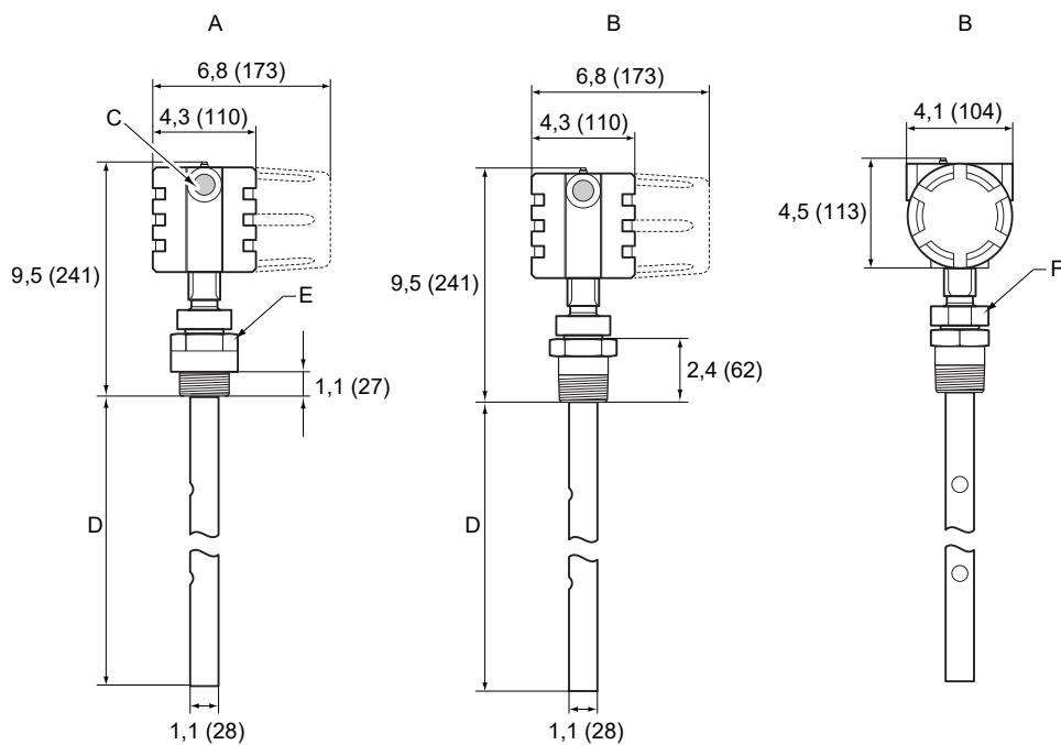
Illustration 29 : Sonde coaxiale avec raccordement fileté
