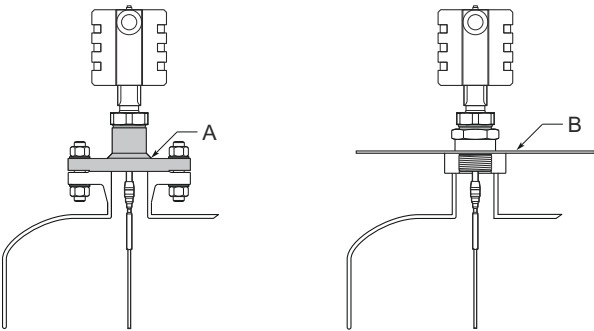
Illustration 20 : Montage dans des réservoirs non métalliques
