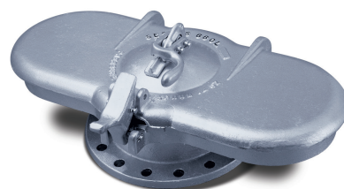
Figure 2. Enardo 660-LB
