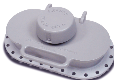
Figure 2. Enardo A-L
